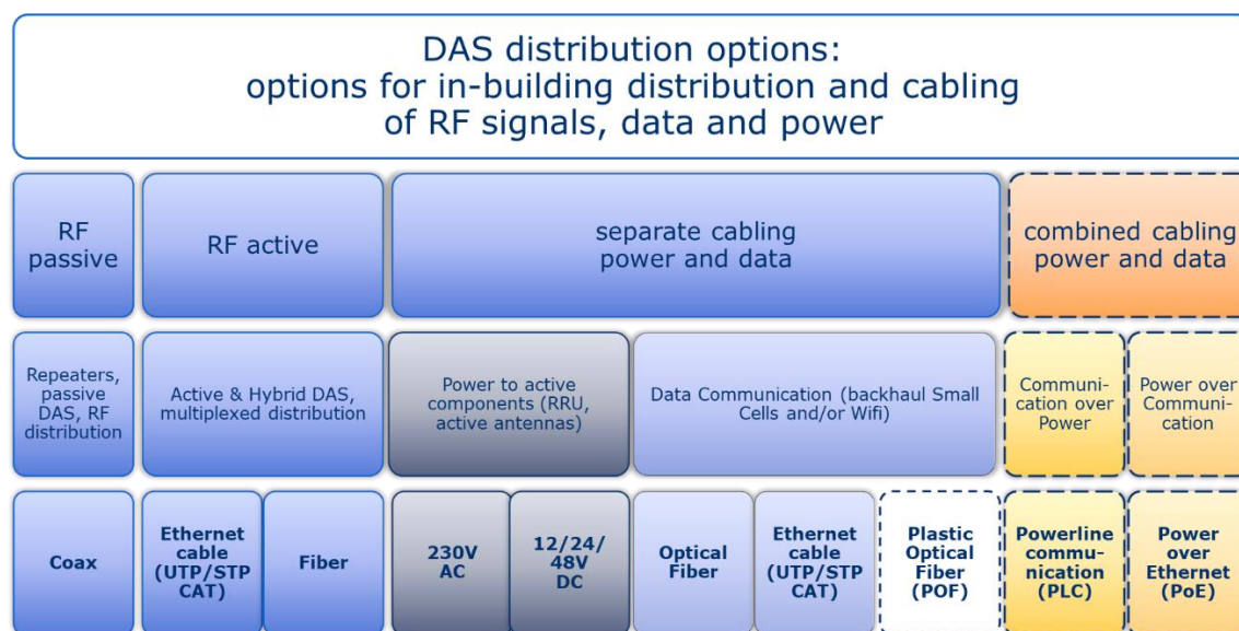
Figuur 23: Verschillende typen passieve infra (kabels) nodig voor in pandige oplossingen
