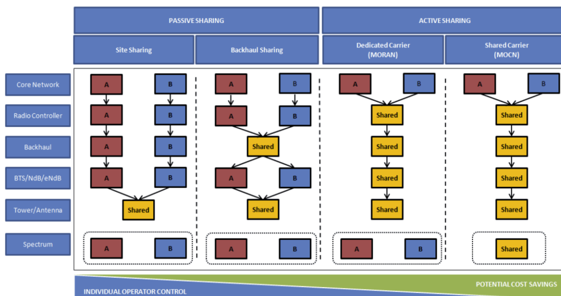
Figuur 20: Verschillende standaarden voor netwerk sharing: (bron: ITU-T / NSN Networks /TMG 48 Niet gedefinieerd door 3GPP maar wordt in de praktijk wel toegepast: MORAN: Multiple Operator Radio Access Network, Gedefinieerd door 3GPP: MOCN = Multi Operator Core Network (bron: ITU-T / NSN Networks /TMGMulti-operator and neutral host small cells, Small Cell Forum)
